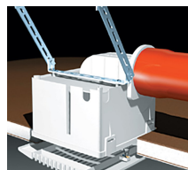
KIT CONTROSOFFITTATORE ORIZZONTALE
